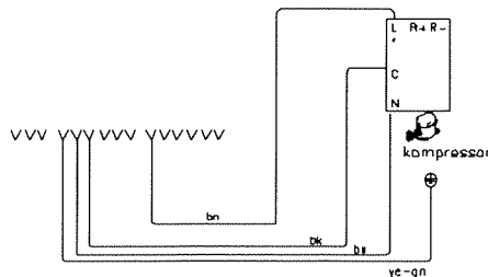
TLV - compressor
