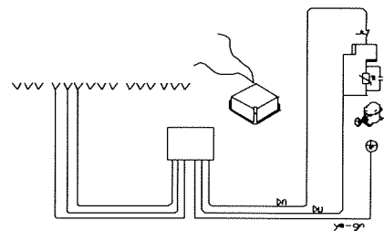
RSD - compressor
